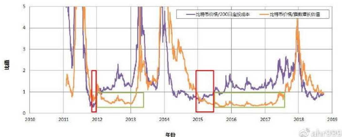
图 3. 比特币价格/200 日定投成本和比特币价格/指数增长估值
