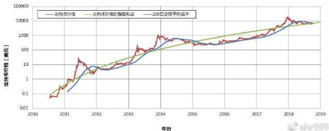
图 2. 比特币历史价格和 200 日定投平均成本
